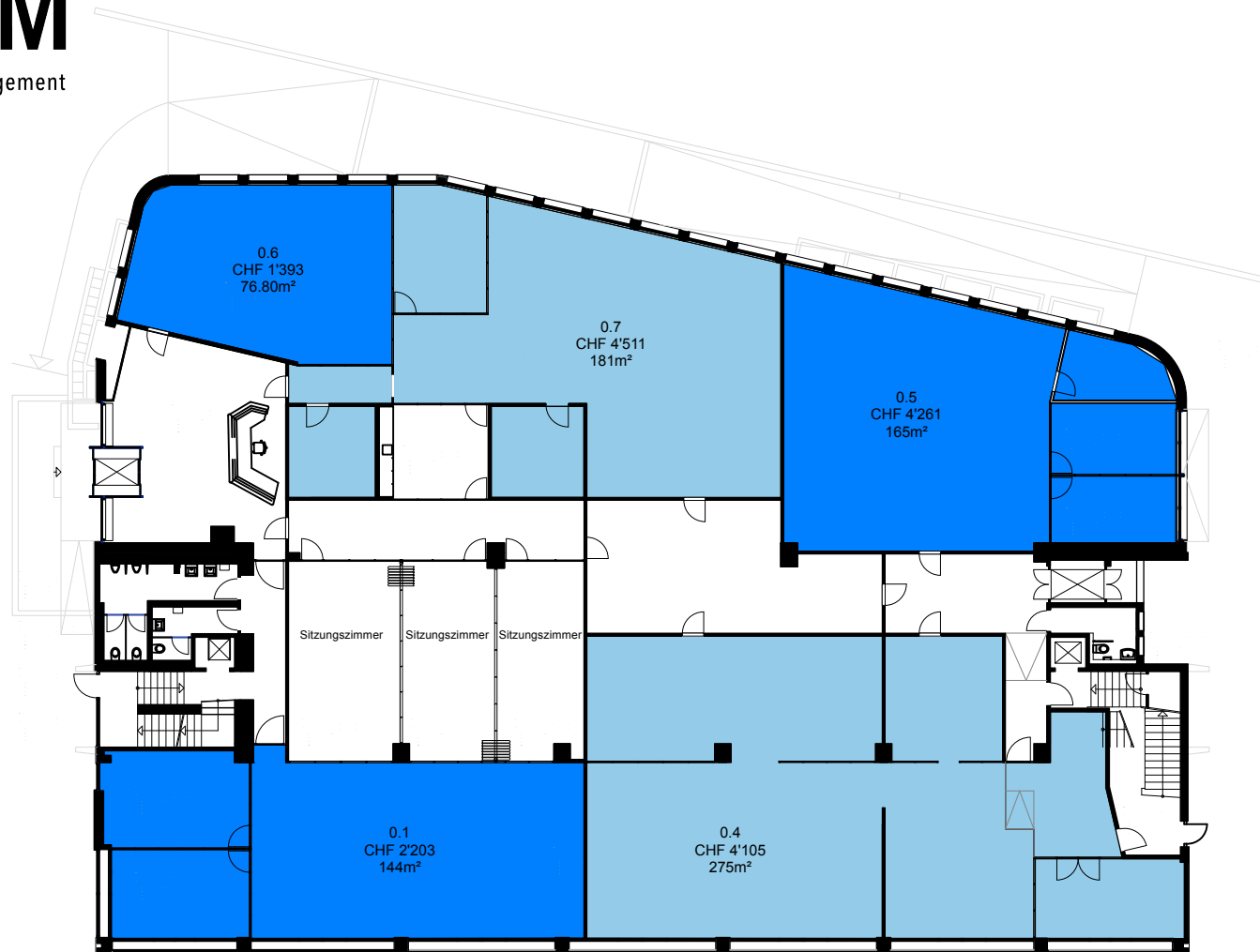
Erdgeschoss Massstab: 1:300
